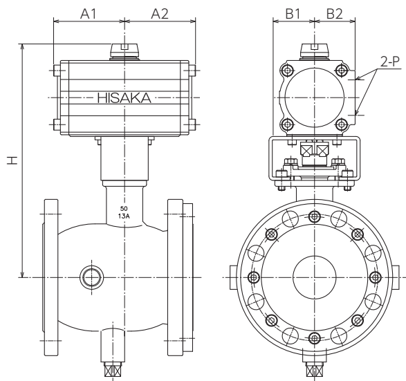
HJ5-AD 複作動アクチュエータ〈JIS10K/150Lb〉
