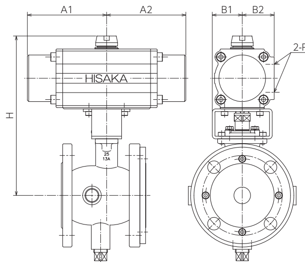
HJ5-AS 単作動アクチュエータ〈JIS10K/150Lb〉
