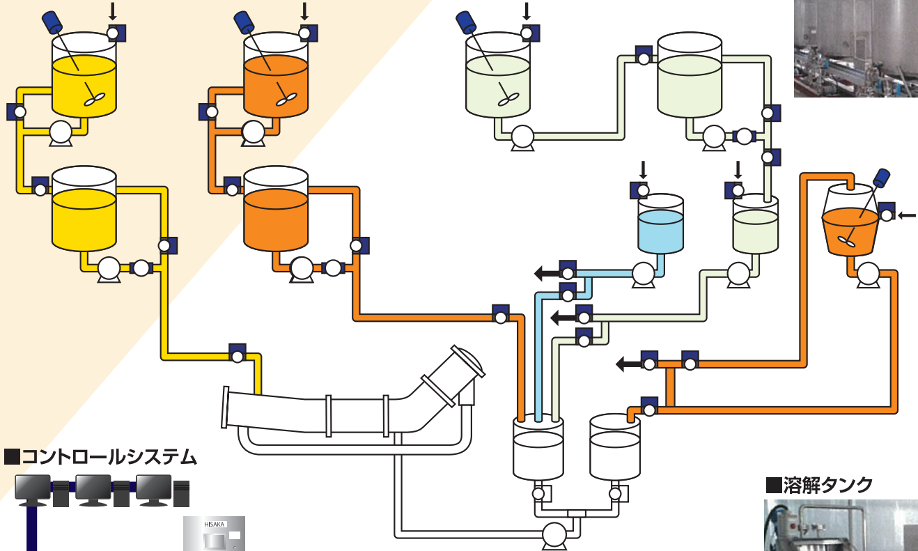
■染料・助剤フロー例
