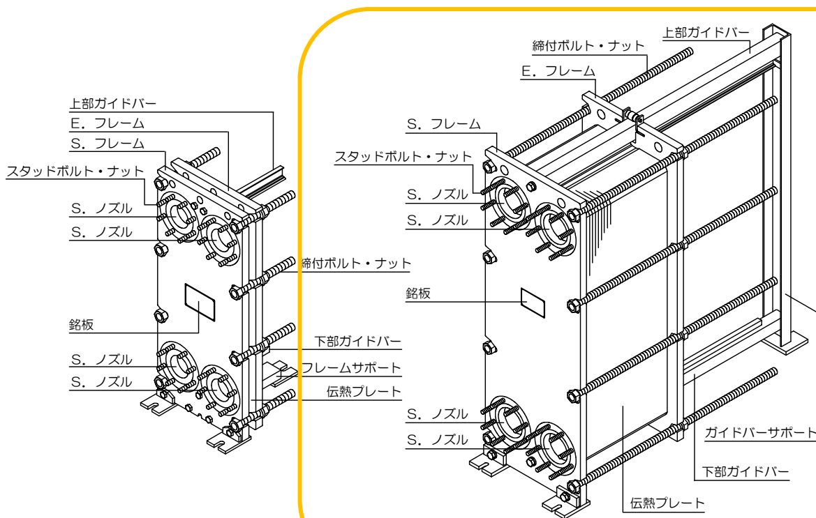
図 2-1 J型熱交換器
