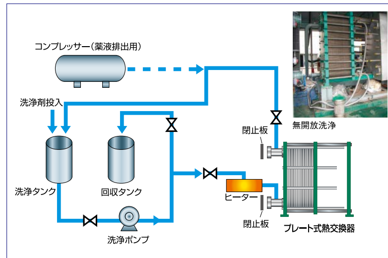
無開放洗浄のフローシート
