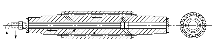
第2図 ドリルドロール
