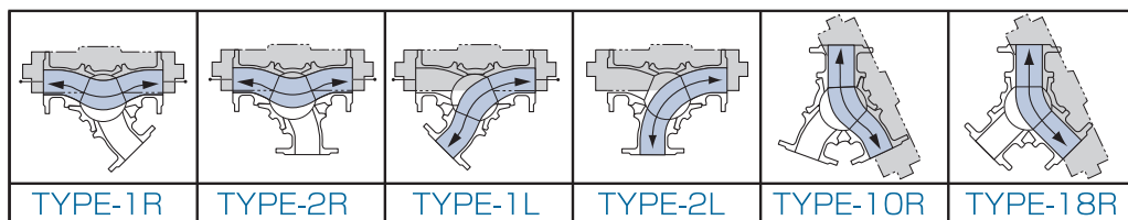
Y型三方弁 組立タイプ
