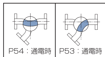
Y型三方弁 通電時流れ方向
