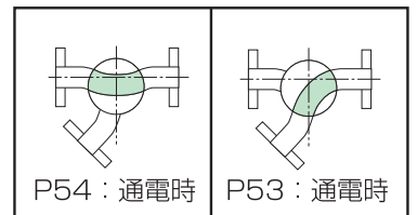
Y型三方弁 通電時流れ方向
