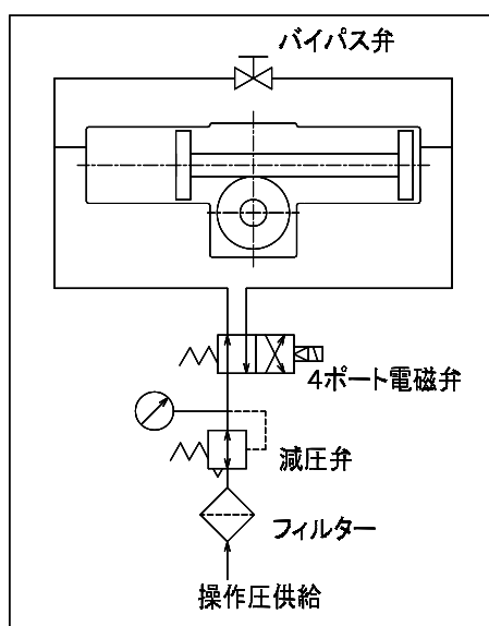
[図3] フローシート
