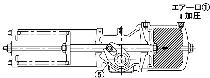
〔図2-A〕エアーク①より加圧
