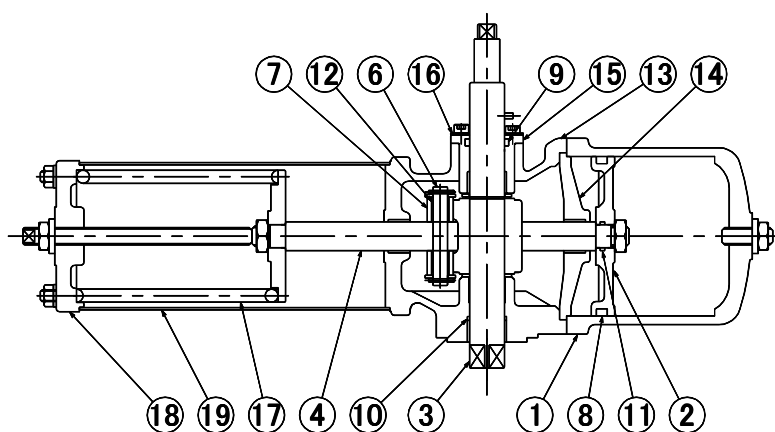
〔図2-A〕エアーク①より加圧
