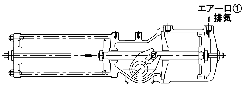
〔図2-B〕エアーク①より排気
