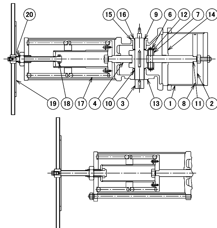
[図4] 単作動型 (TS7H)
