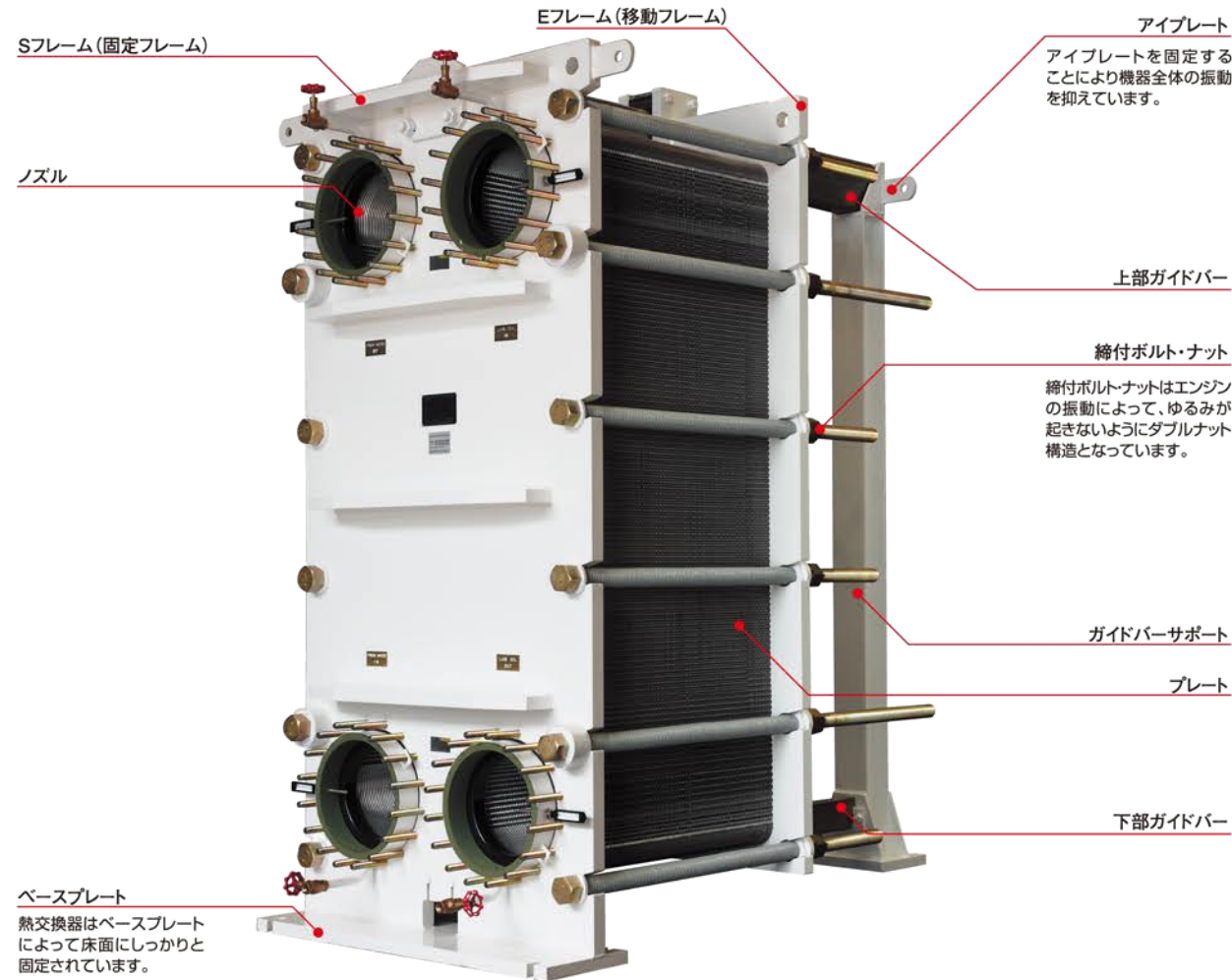
船舶用プレート式熱交換器
