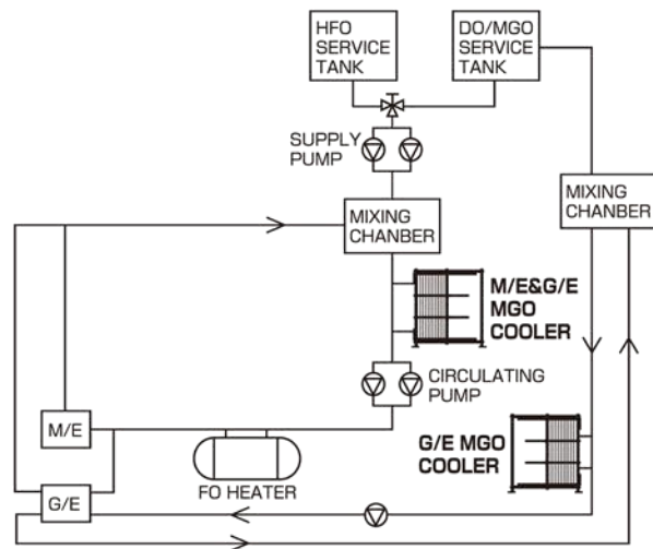
MGO対応プラント燃料油系統フロー図
